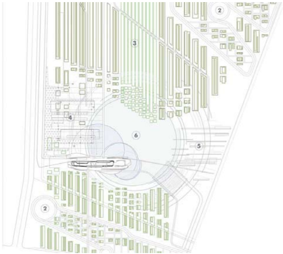
SITUACION / SITE PLAN
