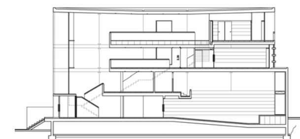
SECCION TRANSVERSAL/ CROSS SECTION
