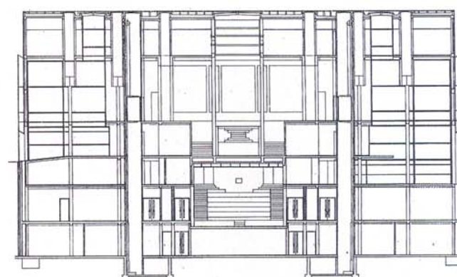
SECCION TRANSVERSAL/ CROSS SECTION
