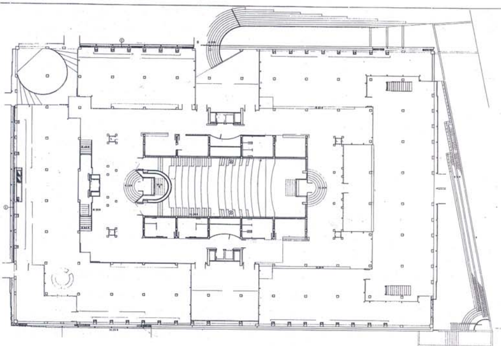
PLANTA DE ACCESO/ GROUND FLOOR
