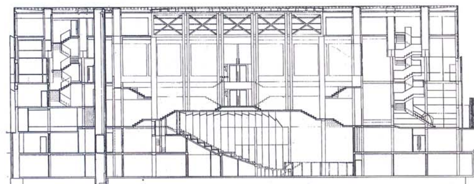
SECCION LONGITUDINAL/ LONGITUDINAL SECTION
