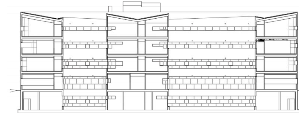
SECCION LONGITUDINAL/ LONGITUDINAL SECTION
