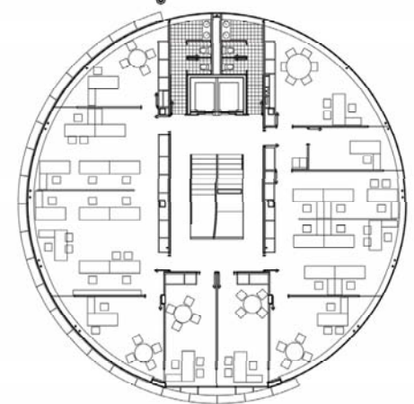
PRIMERA PLANTA/ FIRST FLOOR PLAN
