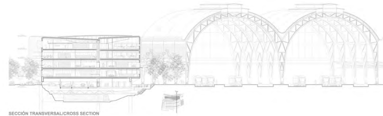
SECCIÓN TRANSVERSAL/CROSS SECTION
