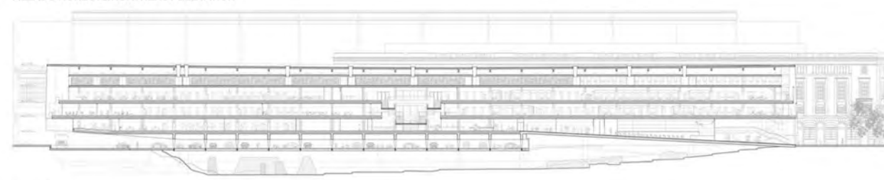
SECCIÓN LONGITUDINAL/LONGITUDINAL SECTION
