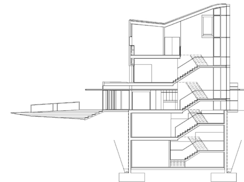
SECCION TRANSVERSAL/ CROSS SECTION
